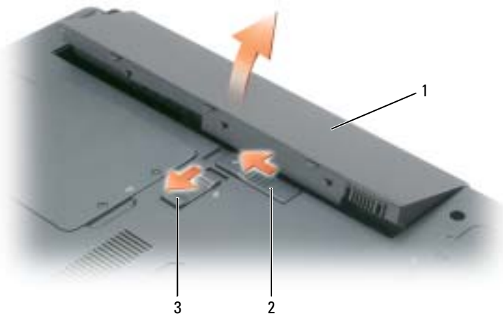
1 电池 2 电池槽释放闩锁 3 电池槽释放闩锁锁
